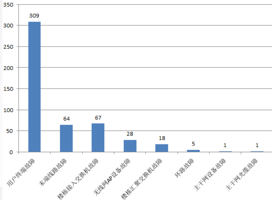
8-12月网络故障原因统计
